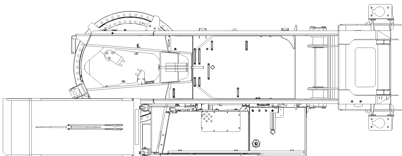
Schnitt B-B
