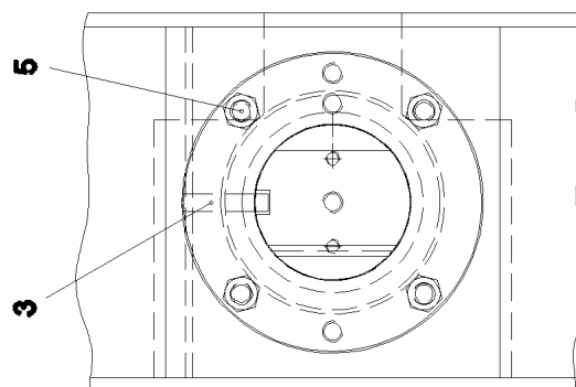
Ansicht Z
